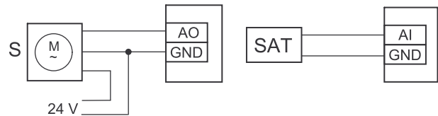
Bild 11 Anbindung Kanalkühlregister
