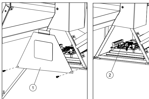
Bild 6 Position der Leiterplatte
