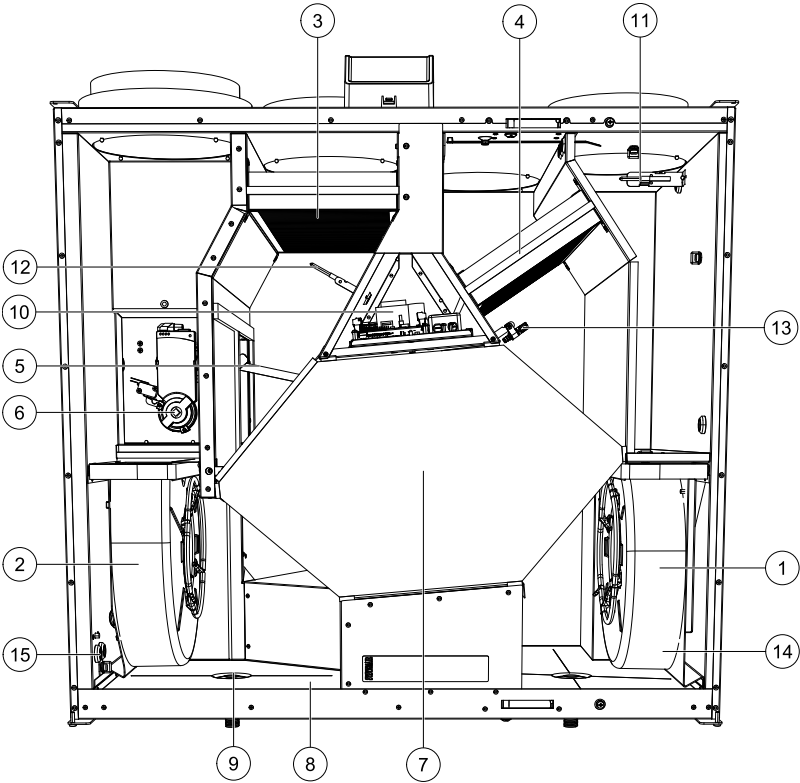
Bild 5 Komponenten
