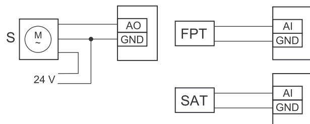
Bild 10 Anbindung Wassernachheizregister
