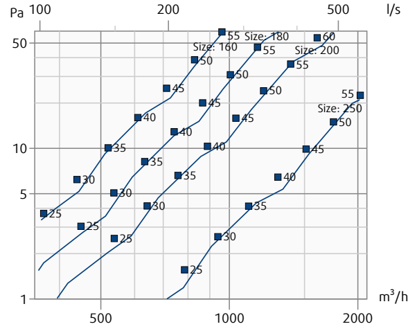
S-RA1-...-B230
