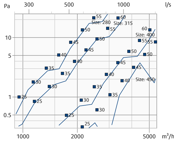
S-RA1-...-B230
