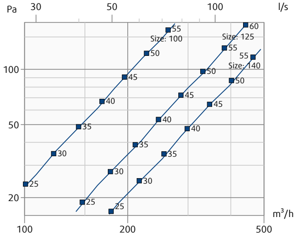
S-RA1-...-B230 + GE1-S-RA1-...-
