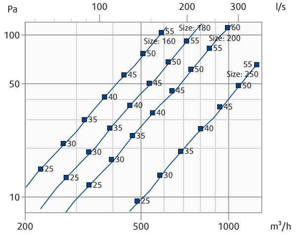
S-RA1-...-B230 + GE1-S-RA1-...-
