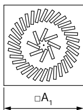
VVKR-A-S-...-40
