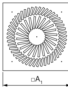
VVKR-A-S-800-72
