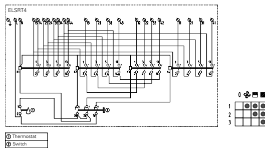
ELSRT4, bedieningskastje met thermostaat, voor 4 units
